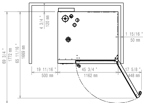
Felülnézet
