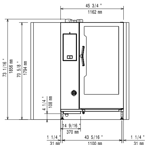
Oldalnézet
